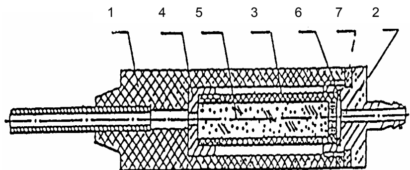
Рисунок 2а– Пробозаборник для модификаций «АВТОТЕСТ-01.03», «АВТОТЕСТ-01.03 ЛТК» и «АВТОТЕСТ-01.04»
